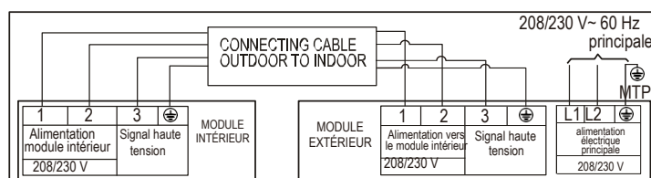
Schéma de connexion (18 K/24K)
